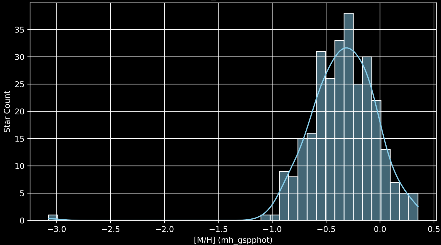
GALAH DR4 Field: [1027] [M/H] (mh_gspphot) (n= 286)
