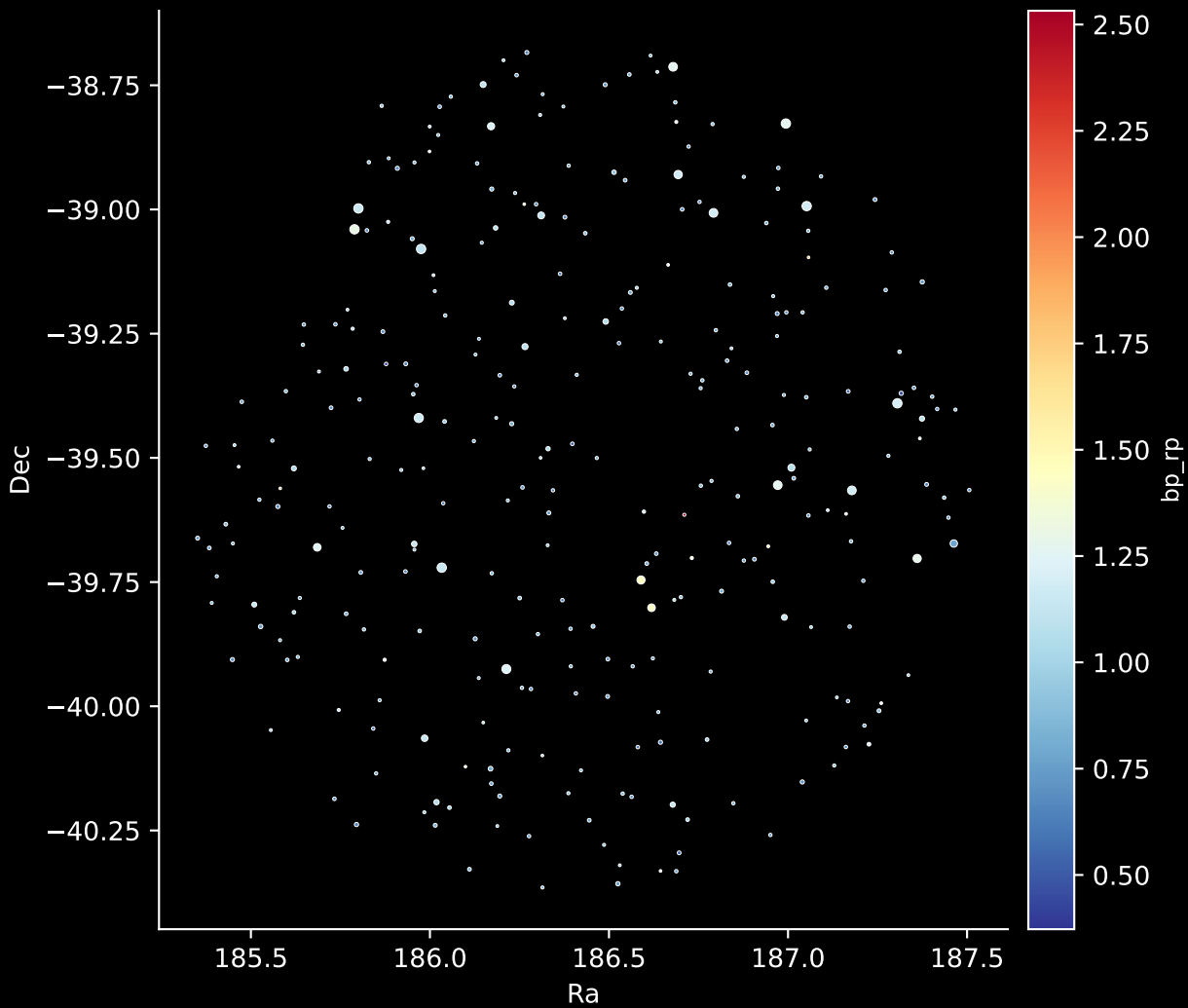
GALAH DR4 Field: [1027] Stars: 287
