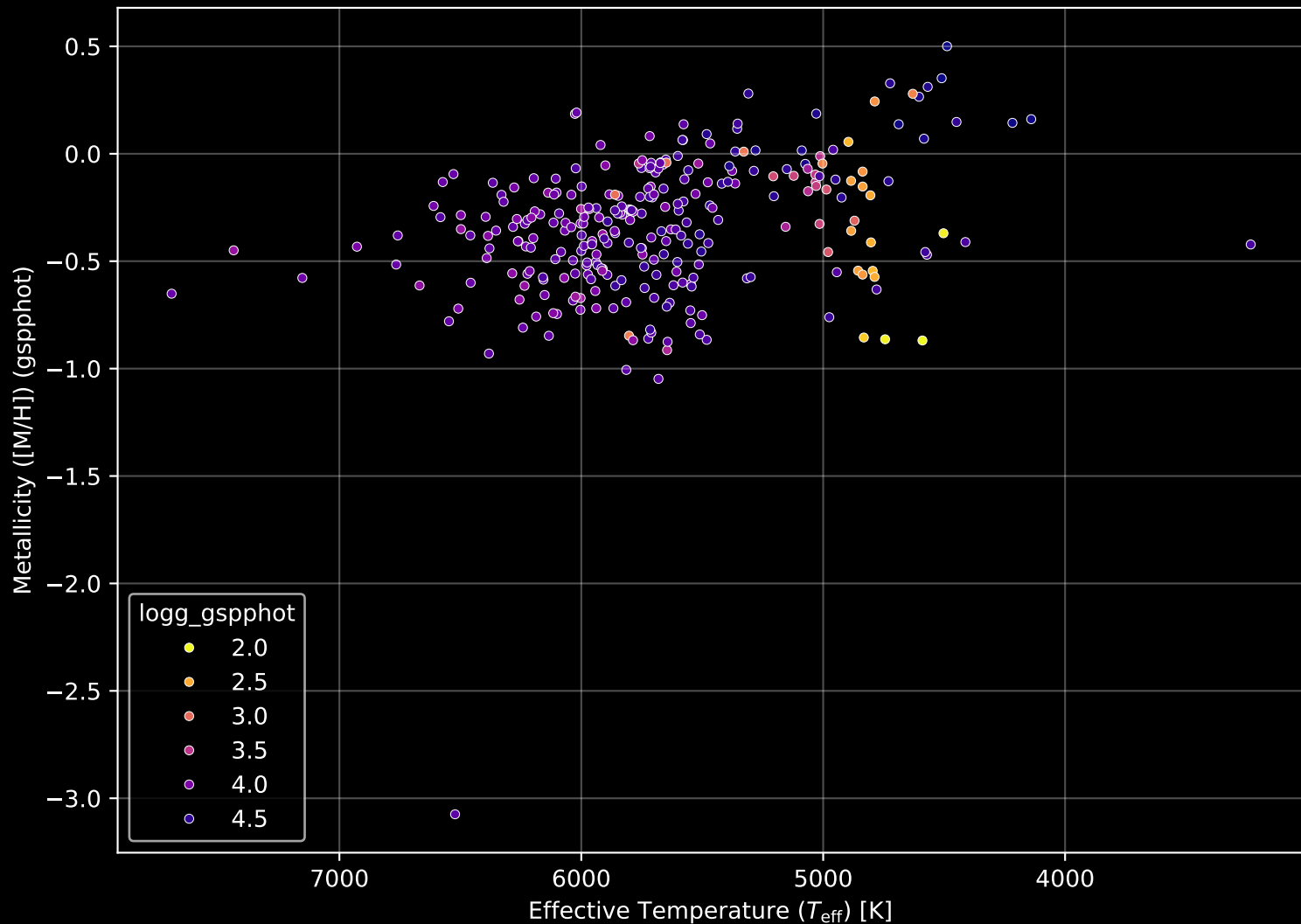
GALAH DR4 Field: [1027] Stellar Population Parameters (n= 287)
