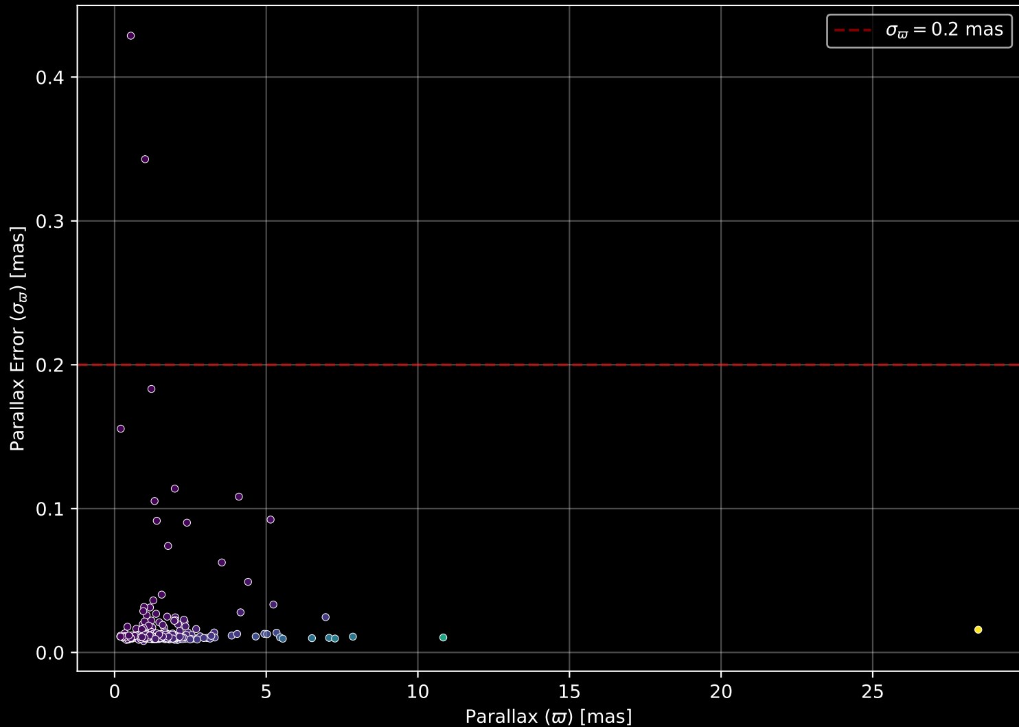
GALAH DR4 Field: [1027] Parallax Quality (n= 287)
